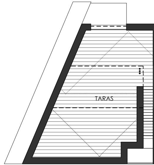
Rzut tarasu na dachu
